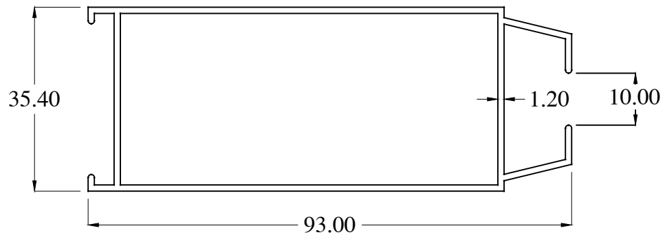
MY1378-D WT : 0.875 Kg/m
