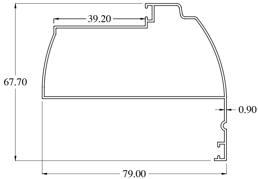
MY1379-C WT : 0.644 Kg/m
