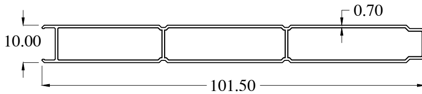
MY1409-C WT : 0.446 Kg/m
