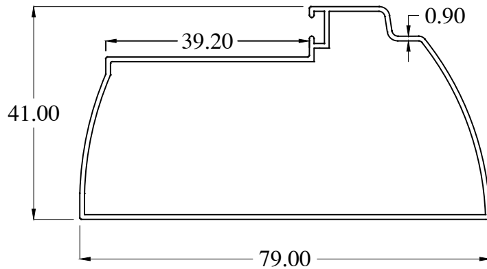
MY1380-C WT : 0.551 Kg/m
