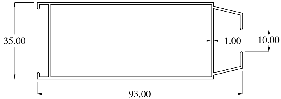
MY1378-C WT : 0.730 Kg/m
