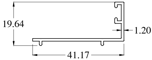
MY1458 WT : 0.227 Kg/m
