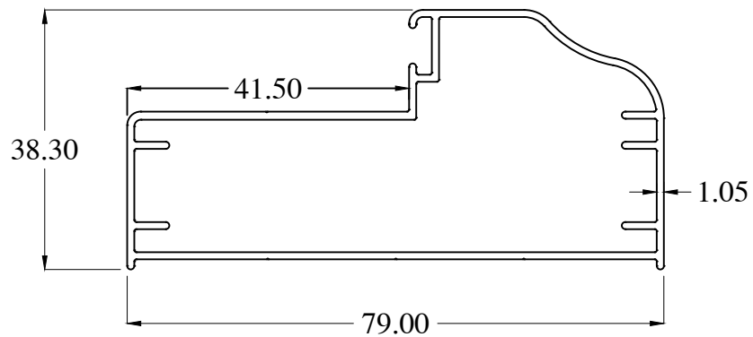
MY1426 WT : 0.735 Kg/m
