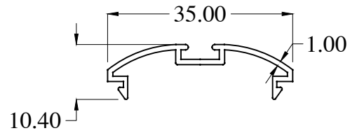
MY1459 WT : 0.165 Kg/m
