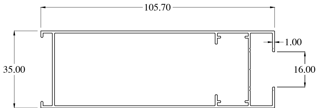
MY1462 WT : 0.839 Kg/m
