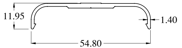
SG1244 WT : 0.313 Kg/m
