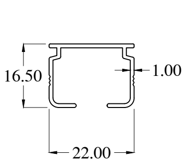
SG1087 WT : 0.175 Kg/m
