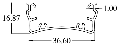
SG1252 WT : 0.267 Kg/m
