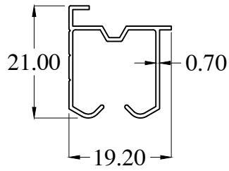
CR1003 WT : 0.144 Kg/m
