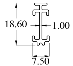
SG1094 WT : 0.119 Kg/m
