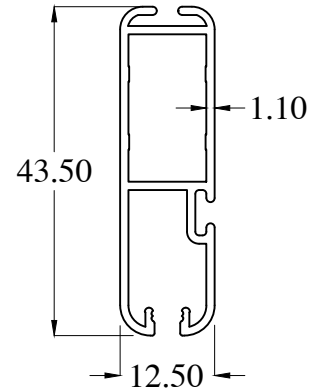
SG1113-1 WT : 0.378 Kg/m
