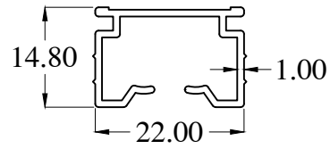
CR1011-1 WT : 0.198 Kg/m
