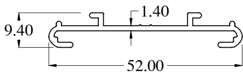
SG1243 WT : 0.307 Kg/m
