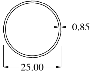
SG1084-1 WT : 0.169 Kg/m
