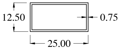
HB0408-1 WT : 0.158 Kg/m
