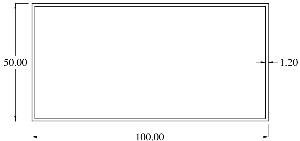
HB1632 WT : 0.960 Kg/m
