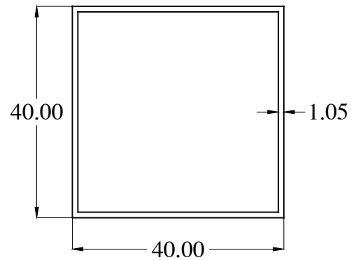
HB1313-1 WT : 0.443 Kg/m
