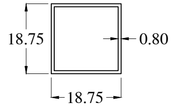
HB0606-1 WT : 0.158 Kg/m
