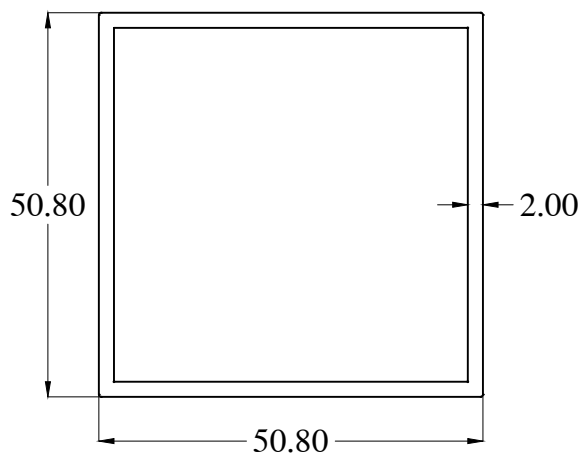
HB1616-2 WT : 1.058 Kg/m
