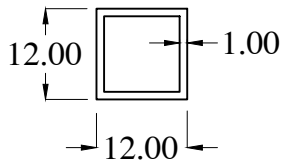
HB0404-1 WT : 0.127 Kg/m
