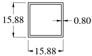
HB0505* WT : 0.131 Kg/m
