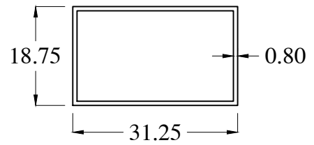
HB0610-1 WT : 0.213 Kg/m
