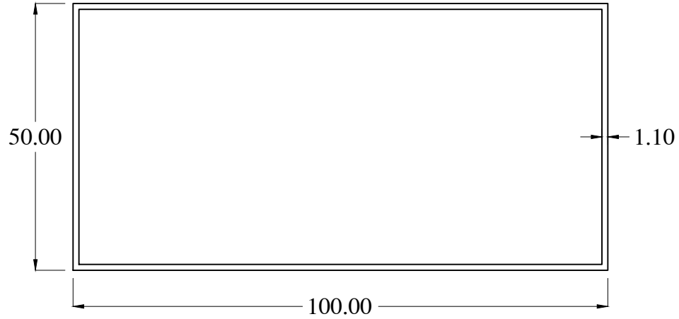
HB1632-1 WT : 0.881 Kg/m
