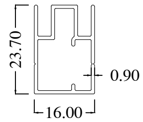
MY1424-A WT : 0.234 Kg/m
