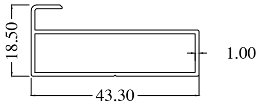
CA2006-C WT : 0.324 Kg/m
