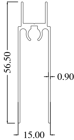
WR1007-1A WT : 0.380 Kg/m
