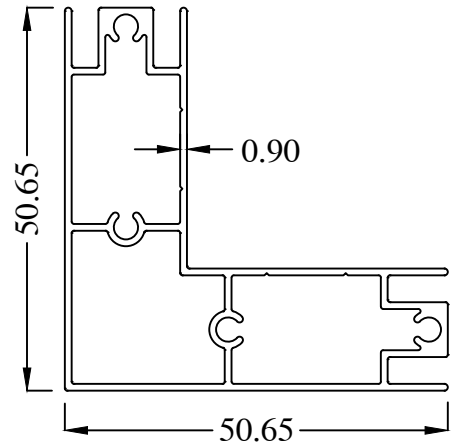
MY1422-A WT : 0.709 Kg/m
