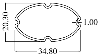
WR1013 WT : 0.249 Kg/m
