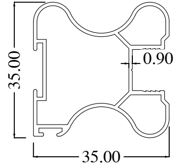
WR1008-A WT : 0.451 Kg/m
