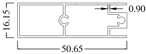
MY1421-A WT : 0.429 Kg/m
