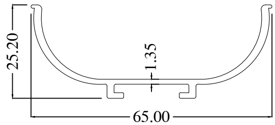
WR1012 WT : 0.468 Kg/m
