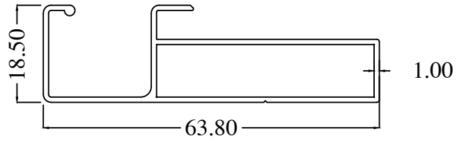
CA2005-C WT : 0.452 Kg/m
