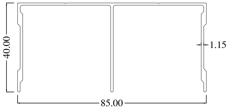
WR1009-B WT : 0.660 Kg/m
