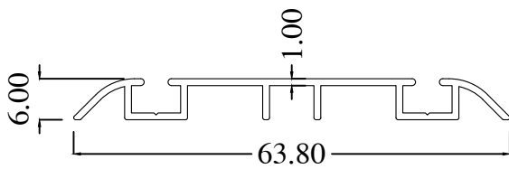
WR1010-A WT : 0.280 Kg/m
