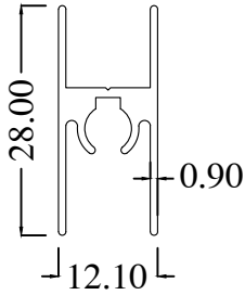
WR1006-1A WT : 0.241 Kg/m
