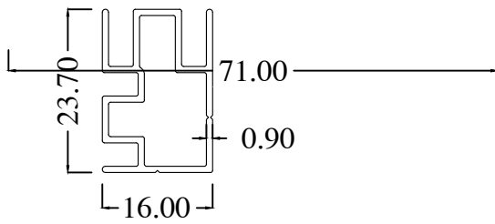
MY1423-A WT : 0.251 Kg/m
