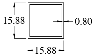
HB0505 WT : 0.131 Kg/m
