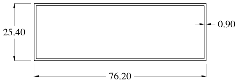
HB0824-3 WT : 0.487Kg/m
