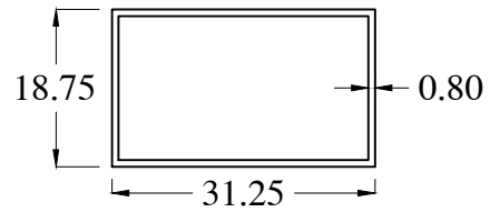
HB0610-1 WT : 0.213 Kg/m
