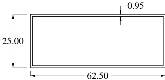
HB0820-1 WT : 0.472 Kg/m
