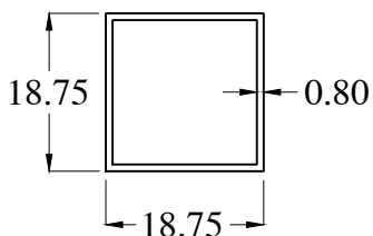
HB0606-1 WT : 0.158 Kg/m
