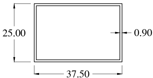
HB0812-1 WT : 0.301 Kg/m
