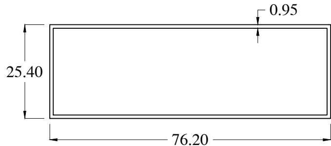
HB0824-2 WT : 0.525 Kg/m
