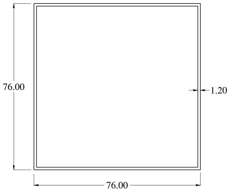
HB2424 WT : 0.976 Kg/m
