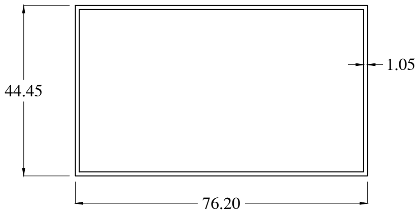
HB1424-1 WT : 0.748 Kg/m
