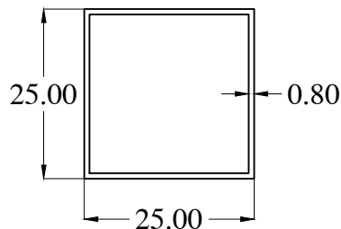
HB0808-1 WT : 0.213 Kg/m
