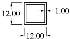
HB0404-1 WT : 0.127 Kg/m
