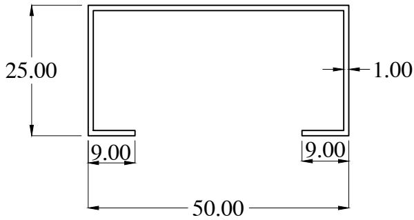
OB0816-1 WT : 0.313 Kg/m
