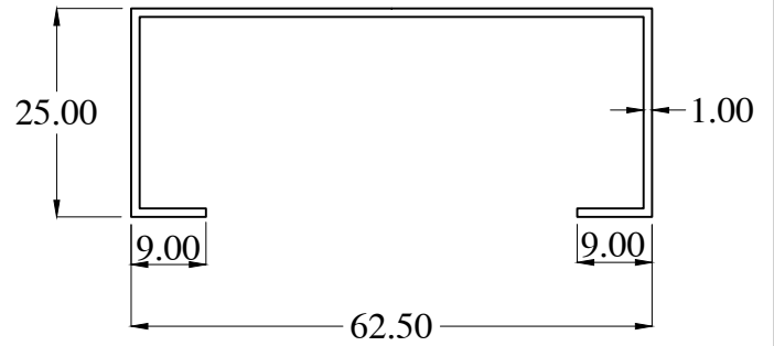
OB0820-1 WT : 0.350 Kg/m
