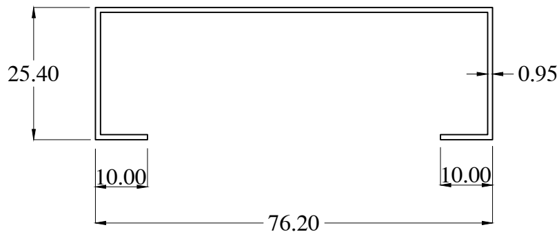
OB0824-2 WT : 0.369 Kg/m
