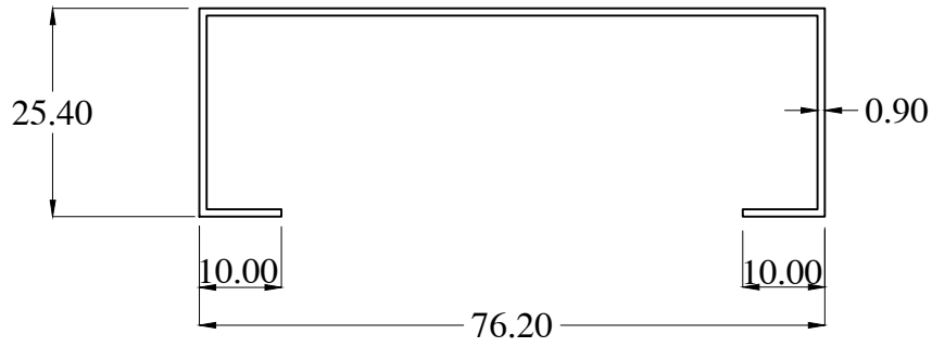
OB0824-4 WT : 0.350 Kg/m
