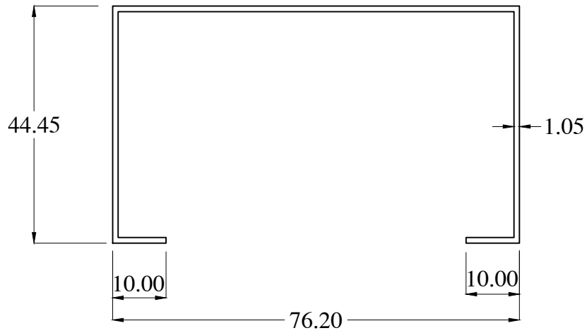
OB1424-1 WT : 0.557 Kg/m
