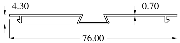
KP5033-1 WT : 0.185 Kg/m
