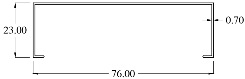
KP5039-1 WT : 0.244 Kg/m
