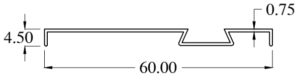
KP1031 WT : 0.160 Kg/m
