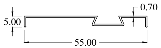
KP1031-1 WT : 0.141 Kg/m
