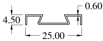
KP1032-2 WT : 0.079 Kg/m
