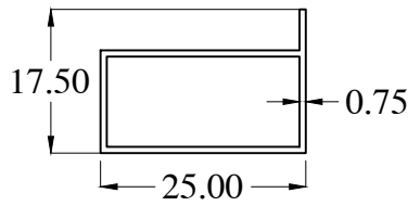
MY1345 WT : 0.169 Kg/m
