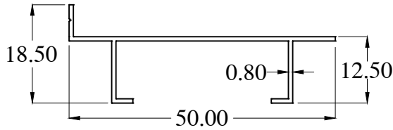
MY1374 WT : 0.199 Kg/m
