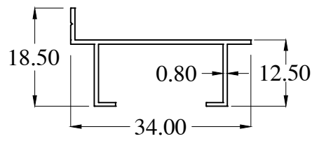
MY1373 WT : 0.149 Kg/m
