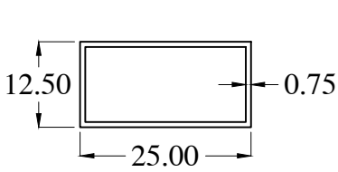
HB0408-1 WT : 0.158 Kg/m
