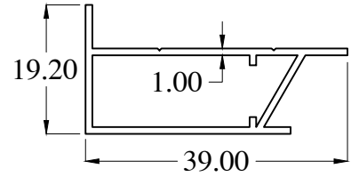
MY1349 WT : 0.276 Kg/m
