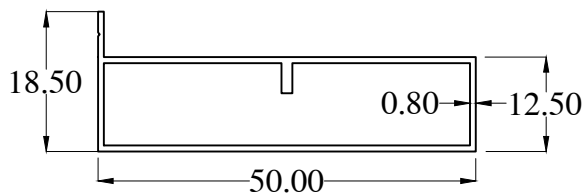
MY1385 WT : 0.292 Kg/m
