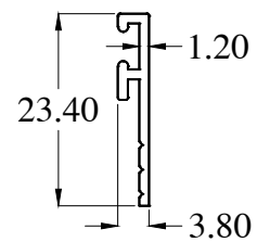
MY1407 WT : 0.105 Kg/m
