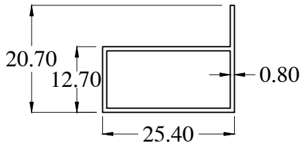
MY1359 WT : 0.176 Kg/m
