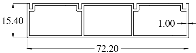
MY1406 WT : 0.563 Kg/m
