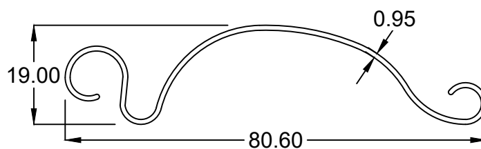
RS 14-1 WT : 0.328 Kg/m
