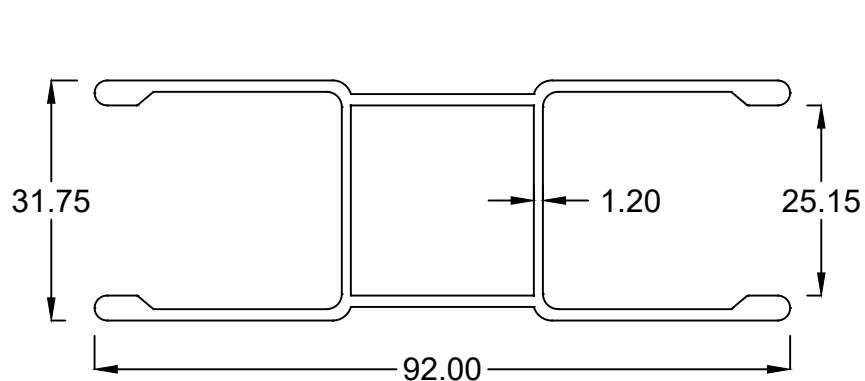
RS11-1 WT : 1.083 Kg/m
