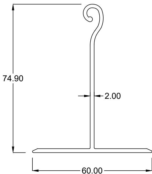
RS13-1 WT : 0.798 Kg/m
