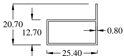
MY1359 WT : 0.176 Kg/m
