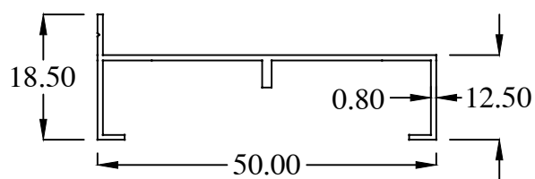
MY1374 WT : 0.199 Kg/m
