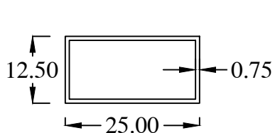
HB0408-1 WT : 0.158 Kg/m
