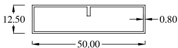
MY1385-A WT : 0.279 Kg/m
